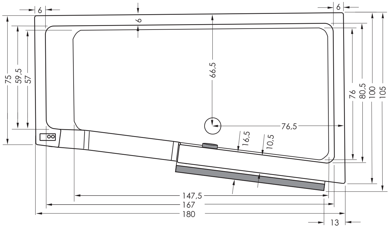
Seitenansicht Standard
