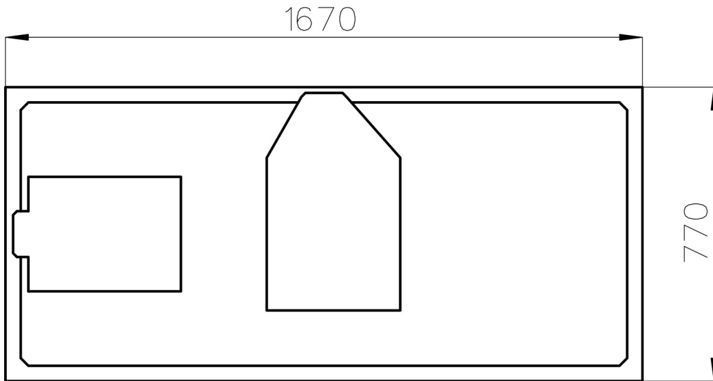
Draufsicht
