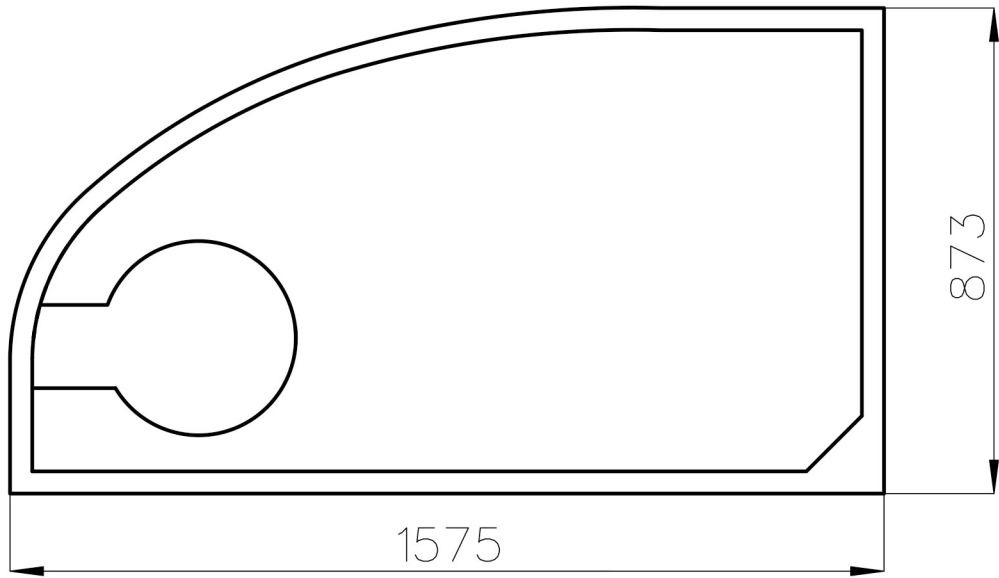
Draufsicht
