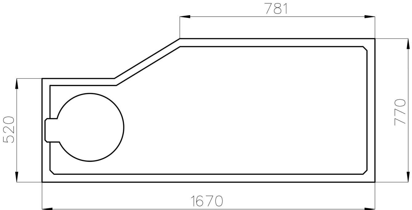
Draufsicht
