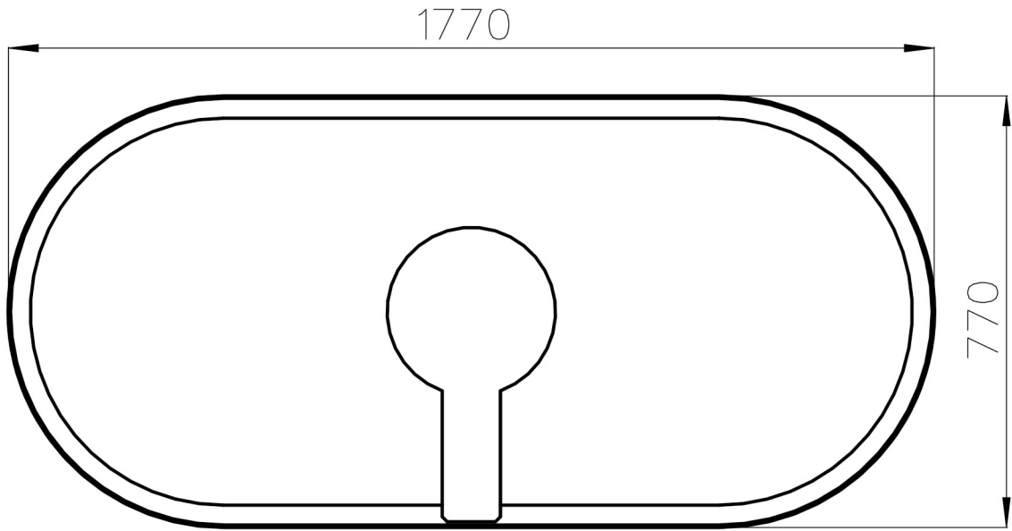
Draufsicht
