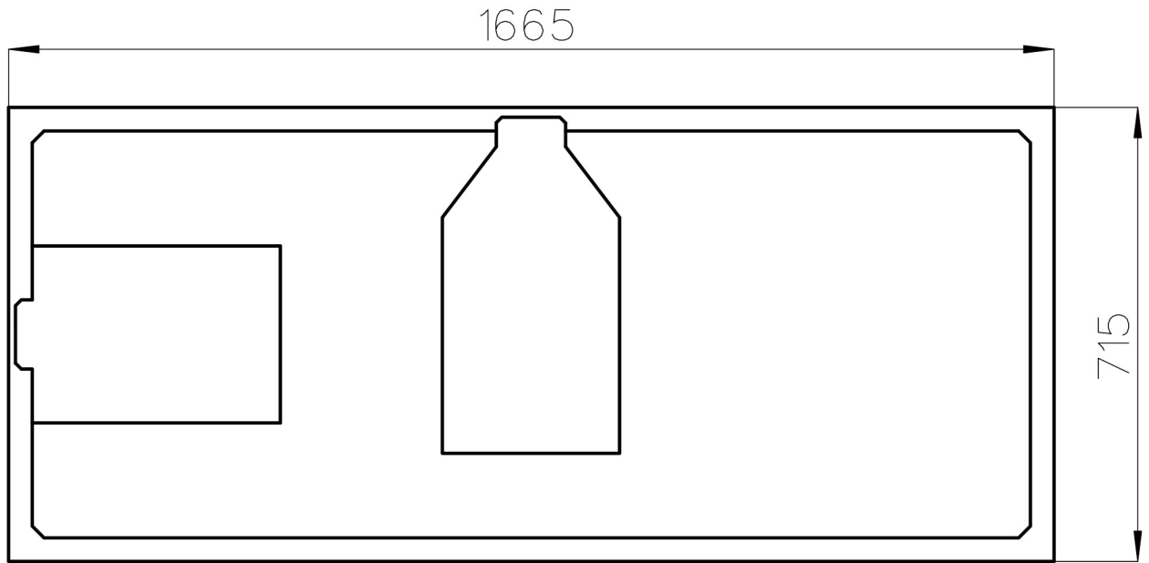
Draufsicht
